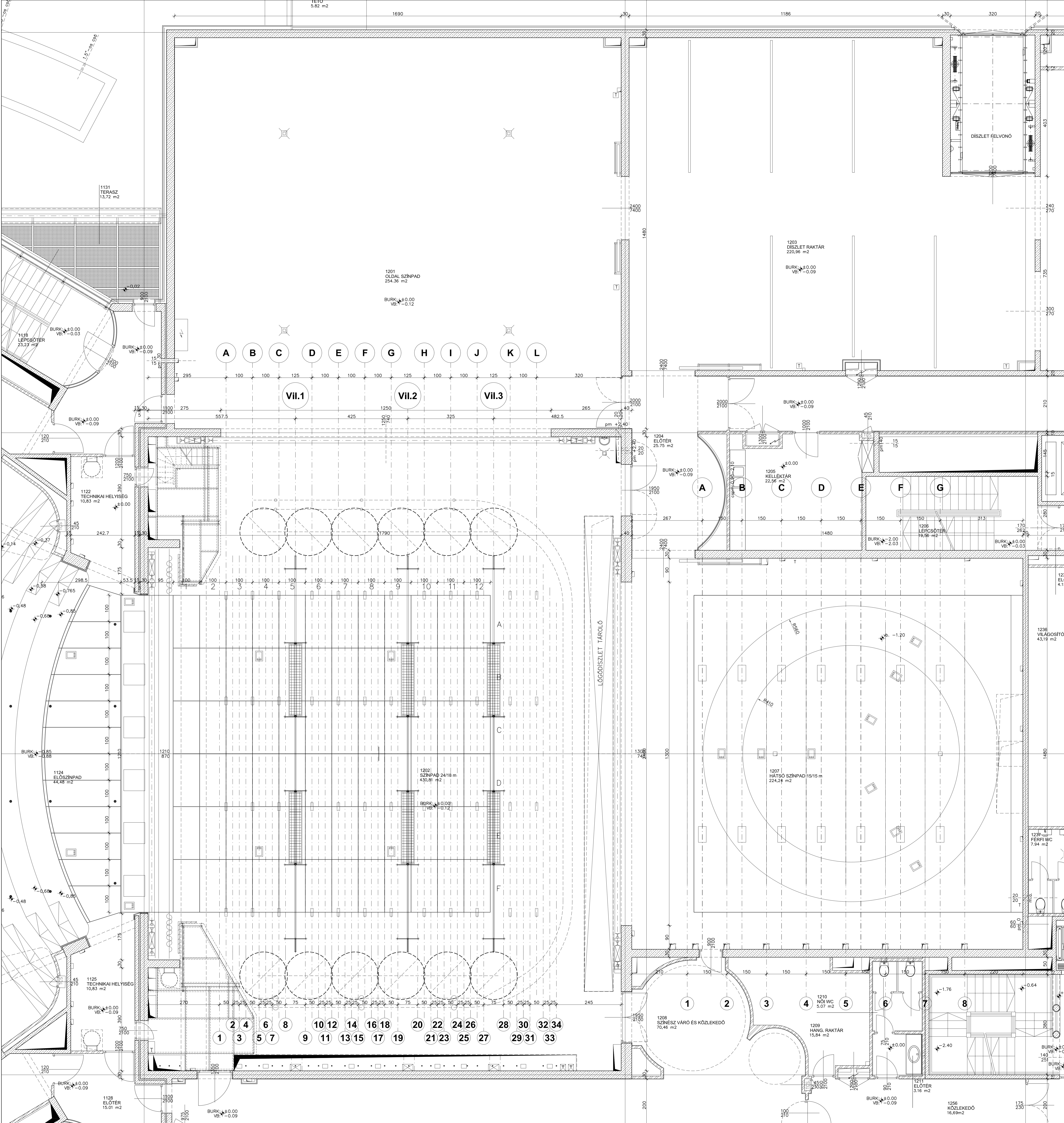
NEMZETI SZÍNHÁZ - SZÍNPAD, HÁTÓSZÍNPAD, OLDALSZÍNPAD I. EMELETI ALAPRAJZA - M = 1 : 50 - 2001. NOVEMBER
